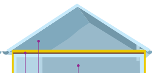
Volume chauffé Espace ventilé non chauffé Isolant avec pare-vapeur ou frein-vapeur
